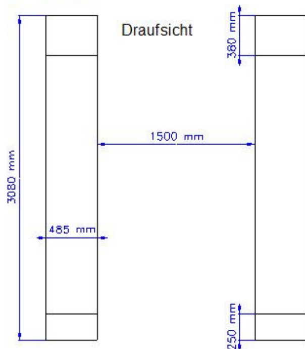
Maße der Fahrspuren auf den WoWa-freecampern
